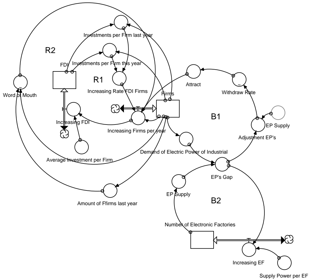
圖 6 中國經濟成長與電力短缺系統模型
