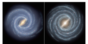
银河系失去两条主臂
