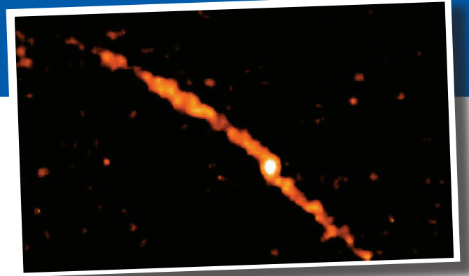
(图为从星团 Palomar 5 (白色斑点) 中出现的恒星分布的彩色编码图; 两条长长的潮汐尾巴 (橙色) 包含了星团质量的 1.3 倍, 并勾勒出它环绕银河系的轨道轮廓。图片来源: SDSS。)
