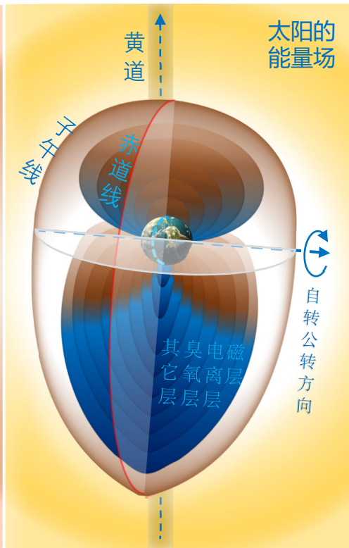
图十七 地球及其能量场示意图
