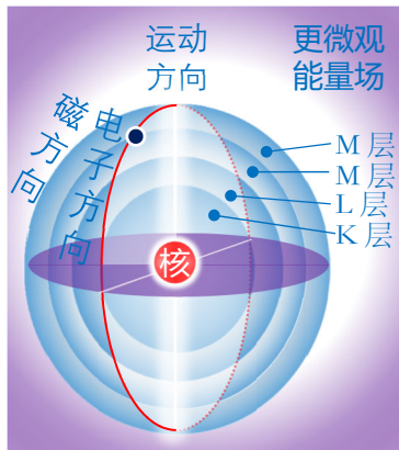
图十三 原子及其能量场示意图
