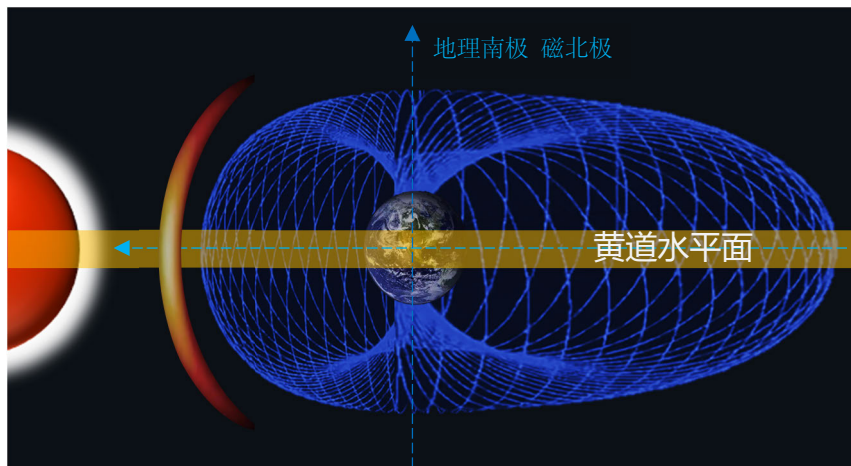
图十一 太阳能量场时空中，地球空间的磁场示意图
