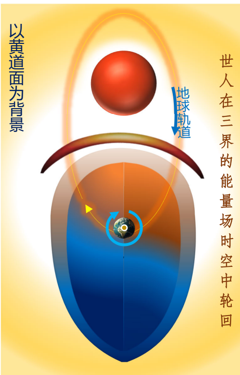
图二五 黄道平面的地球能量场 (看同一层次)
